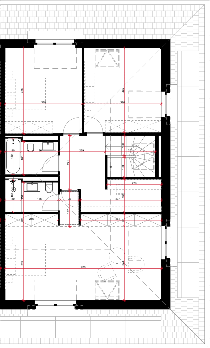
Niveau Combles
